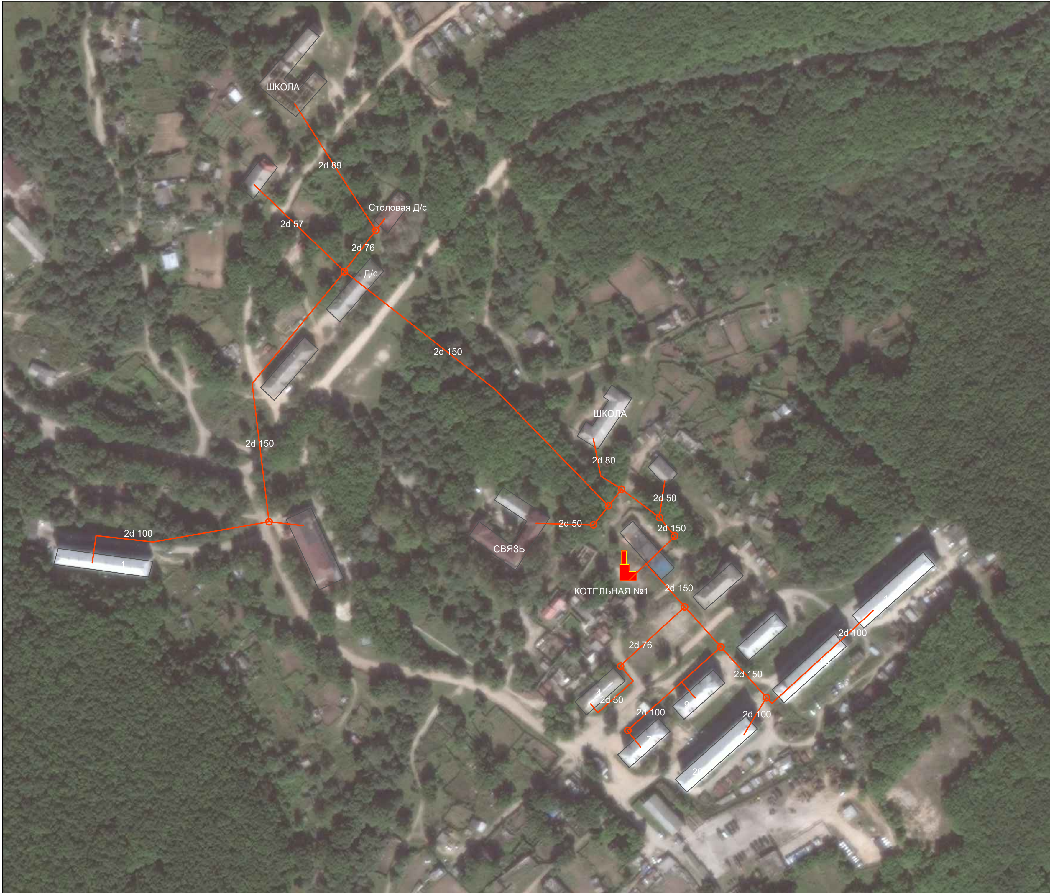
Схема теплоснабжения с. Тимофеевка, котельная №1 фрагмент территории
